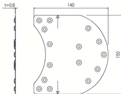
リブレースプレート
