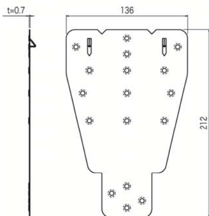
ターミネーションプレート
