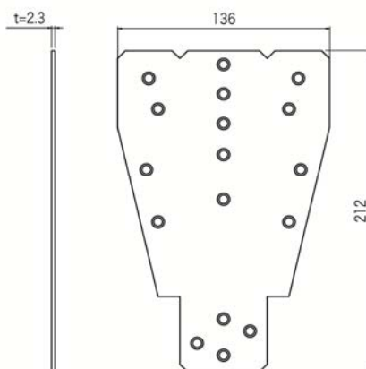
ブレースプレート I
