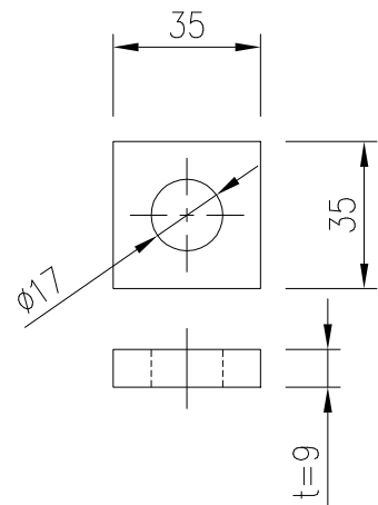
専用角座金
