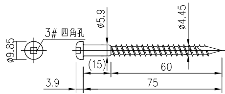
たて枠側 YS-N75(ブラック): 6本
