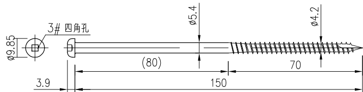
横架材側 YS-N150(シルバー): 4本
