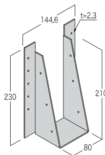
■ 製品図
