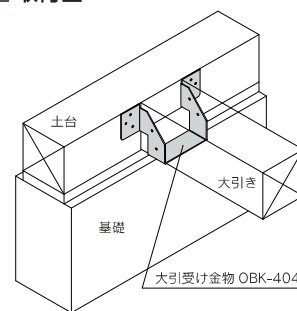
■ 取付図
