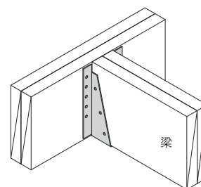
■ 取付図
