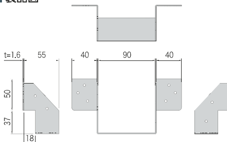
■ 製品図
