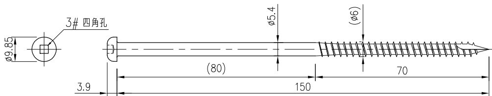
横架材側 YS-N150(シルバー): 2本
