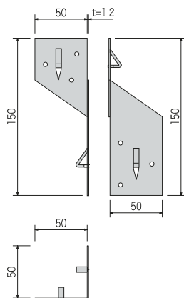
■ 製品図
