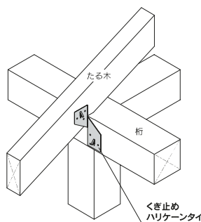
■ 取付図
