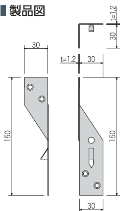
■ 製品図
