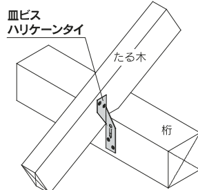
■ 取付図
