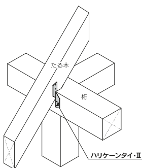
■ 取付図
