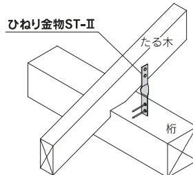
■ 取付図
