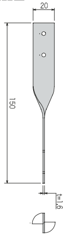
■ 製品図
