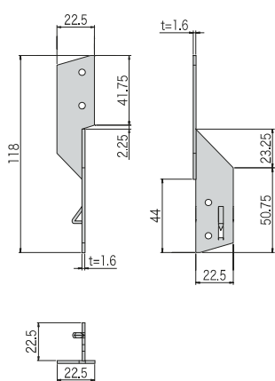
■ 製品図
