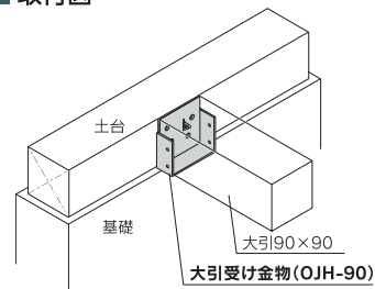
■ 取付図
