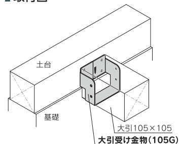
■ 取付図
