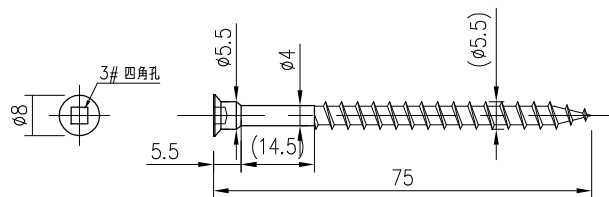
横架材側ビス YA-S75(ブラック): 4本
