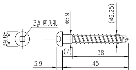
柱側 YD-N45(シルバー): 5本
