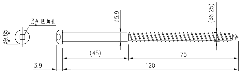
横架材側 YD-N120(シルバーレッド): 2本
