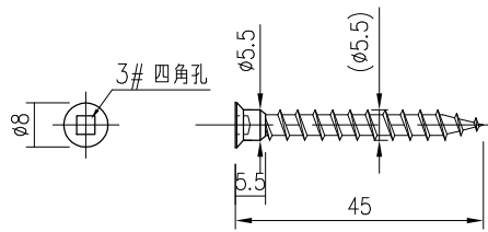
柱・横架材側 YA-S45(シルバー) : 12本
