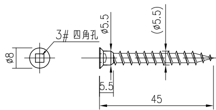
柱・横架材側 YA-S45(シルバー) : 9本
