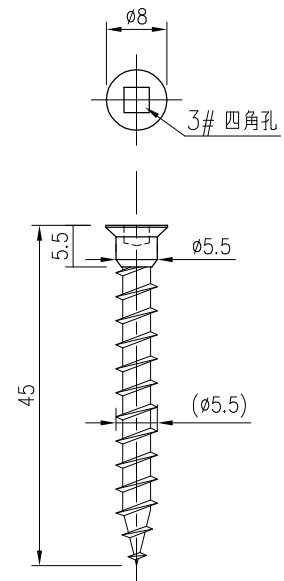
柱・横架材側 YA-S45(シルバー) : 6本
