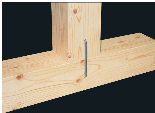
■ 施工例
