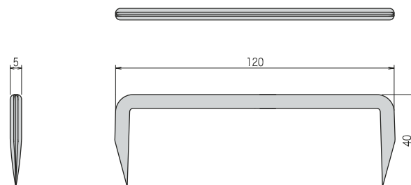
■ 製品図
