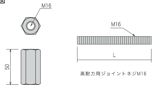
高耐力用ロングナットM16×50
