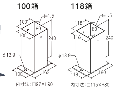
内寸法: □97×H90
