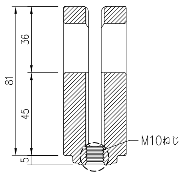
断面 B-B
